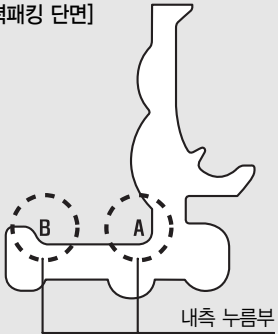
[압력패킹 단면]
